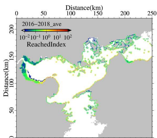
図 1-イ-b-7 各海域における放出粒子数が一定と仮定した場合の着底ポテンシャル指数(1～3 月、3年間平均)
