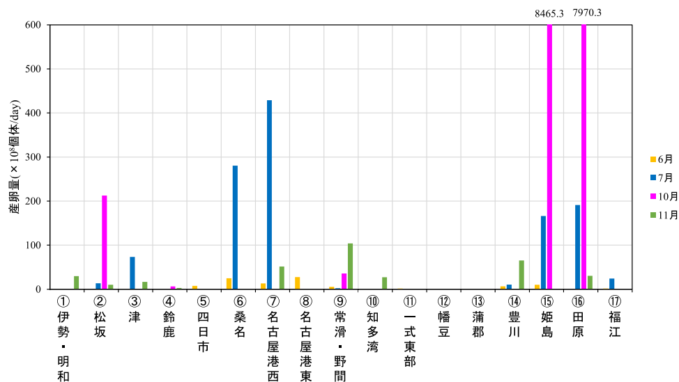
図 1-ア-b-8 孵化後 24 時間～7 日（浮遊条件 a）の粒子追跡計算の解析結果より求めた各放水区における推定産卵量の一覧
