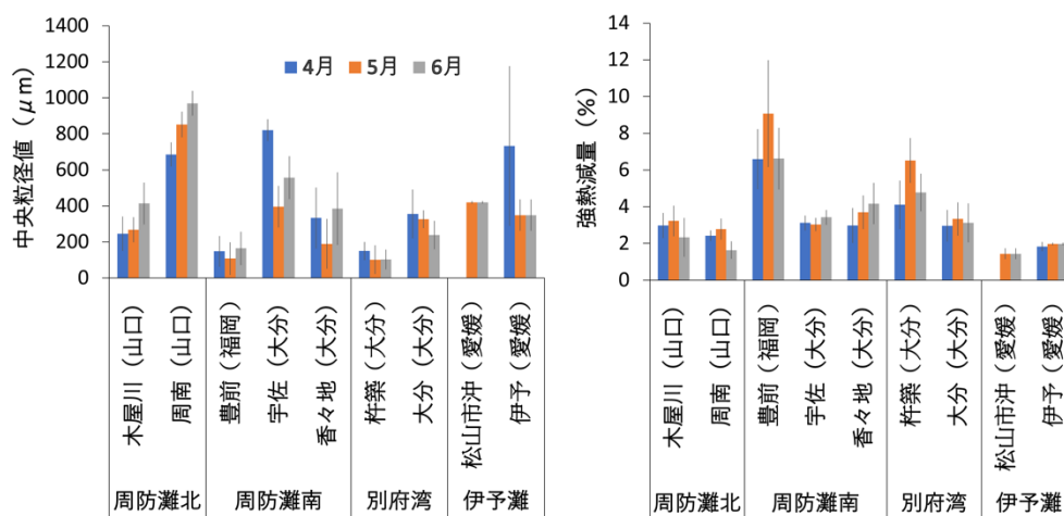
図 1-イ-a-6. 各種魚調査地区における月ごとの調査地点の中央粒径値および強熱減量の平均値 (±標準誤差)
