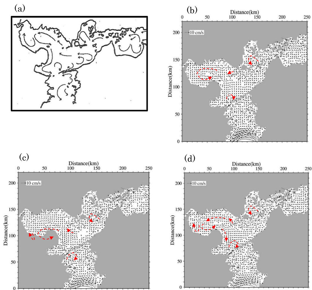
図1-イ-b-3 平均流分布図。(a)瀬戸内海表層における恒流模式図(柳・樋口、1979)。(b)2016年1月、(c)2017年1月、(d)2018年1月における月平均流速分布(全層平均、モデル結果)
