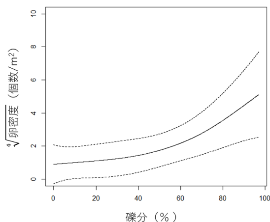
図 2-イ-1. マコガレイの卵数と礫分(粒径 1.0mm 以上)の関係。実線は卵数の推定値、点線に挟まれた領域はその推定値のばらつきの範囲
