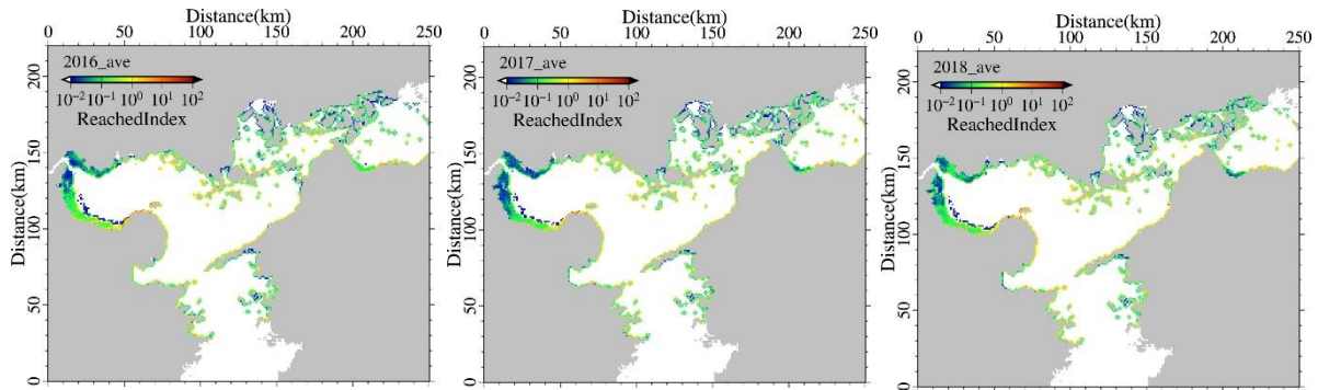
図1-イ-b-6 各海域における放出粒子数が一定と仮定した場合の着底ポテンシャル指数 (左図：2016年1～3月、中図：2017年1～3月、右図：2018年1～3月)
