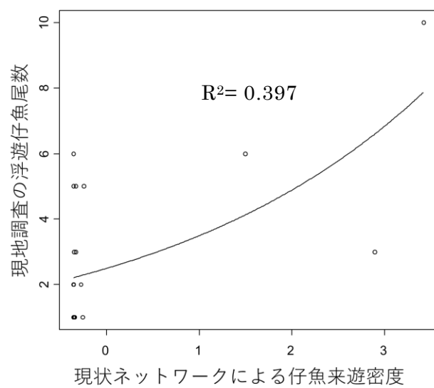
図 1-イ-b-11 現地調査の浮遊仔魚尾数と数値解析の現状ネットワークの仔魚来遊密度（尾数/m³を標準化）との関係
