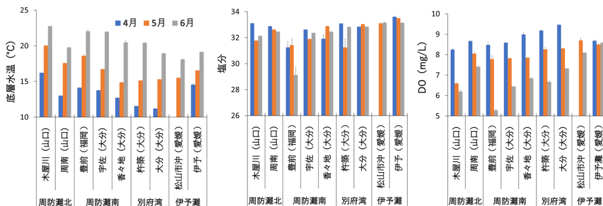
図 1-イ-a-5. 各種魚調査地区における月ごとの底層水温、底層塩分、底層 DO の平均値 (±標準誤差)
