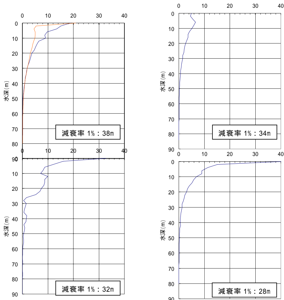
図65 相対光量子の鉛直分布
