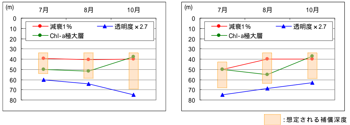
図 58 想定される補償深度帯 (左 : St.1、右 : St.2) (相対光量子減衰 1%・透明度×2.7・Chl-a 極大層)
