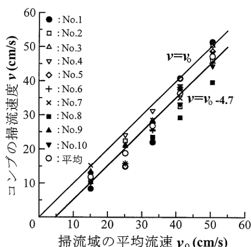
図 11 コンブの掃流速度
