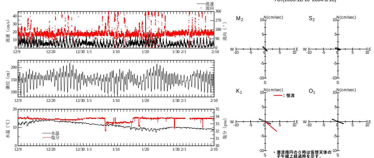
図 15 冬期流況 (左: 時系列図 流向・流速, 潮位, 水温・塩分, 右: 潮流楕円図 上 M 2 , S 2 , 下 K 1 , O 1 )
