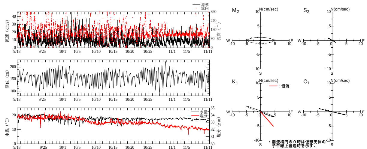
図 14 秋期流況 (左: 時系列図 流向・流速, 潮位, 水温・塩分, 右: 潮流楕円図 上 M 2 , S 2 , 下 K 1 , O 1 )
