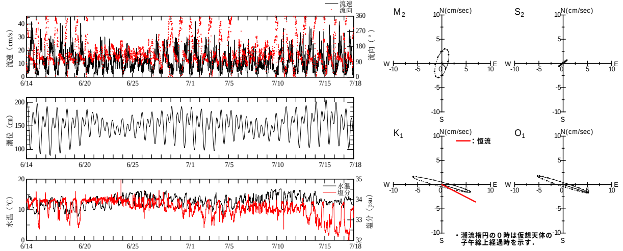
図 13 夏期流況 (左: 時系列図 流向・流速, 潮位, 水温・塩分, 右: 潮流楕円図 M 2 , S 2 , 下 K 1 , O 1 )
