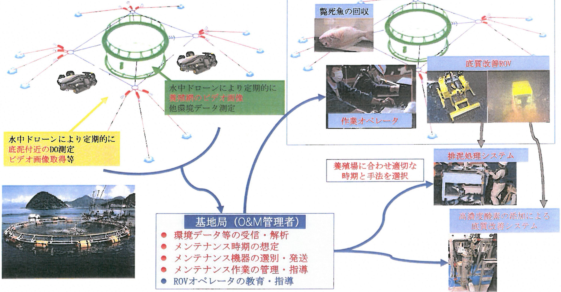
図4 水中ドローンを用いたオペレーション&メンテナンスシステムによる持続的な養殖生産の推進
