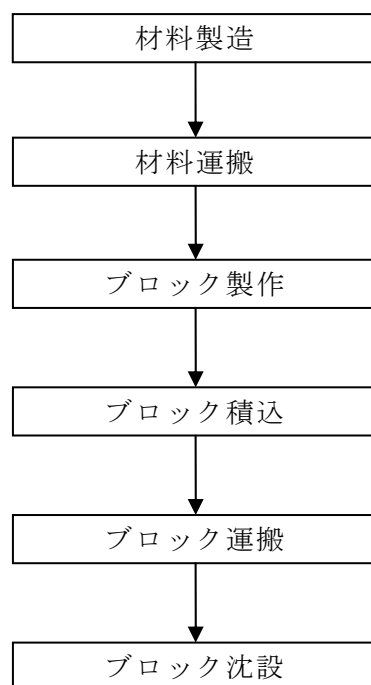
図VI-4.2.1 施工フロー
