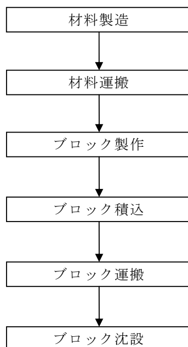
図VI-4.2.5 施工フロー
