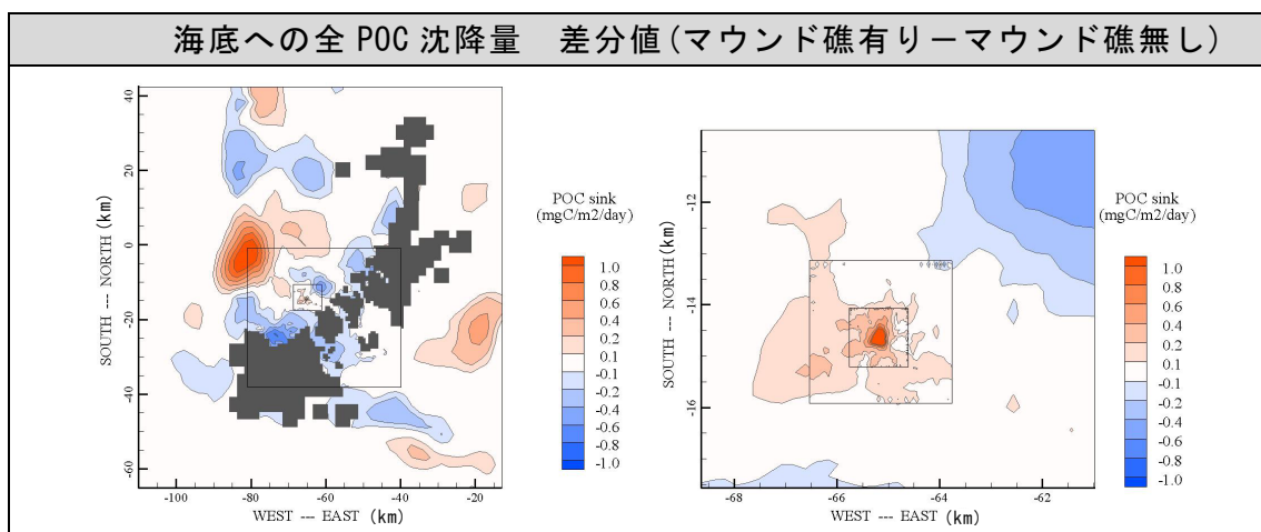
図VI-4. 3. 15 海底への全 POC 沈降量差分値 (マウンド礁有リーマウンド礁無し)
