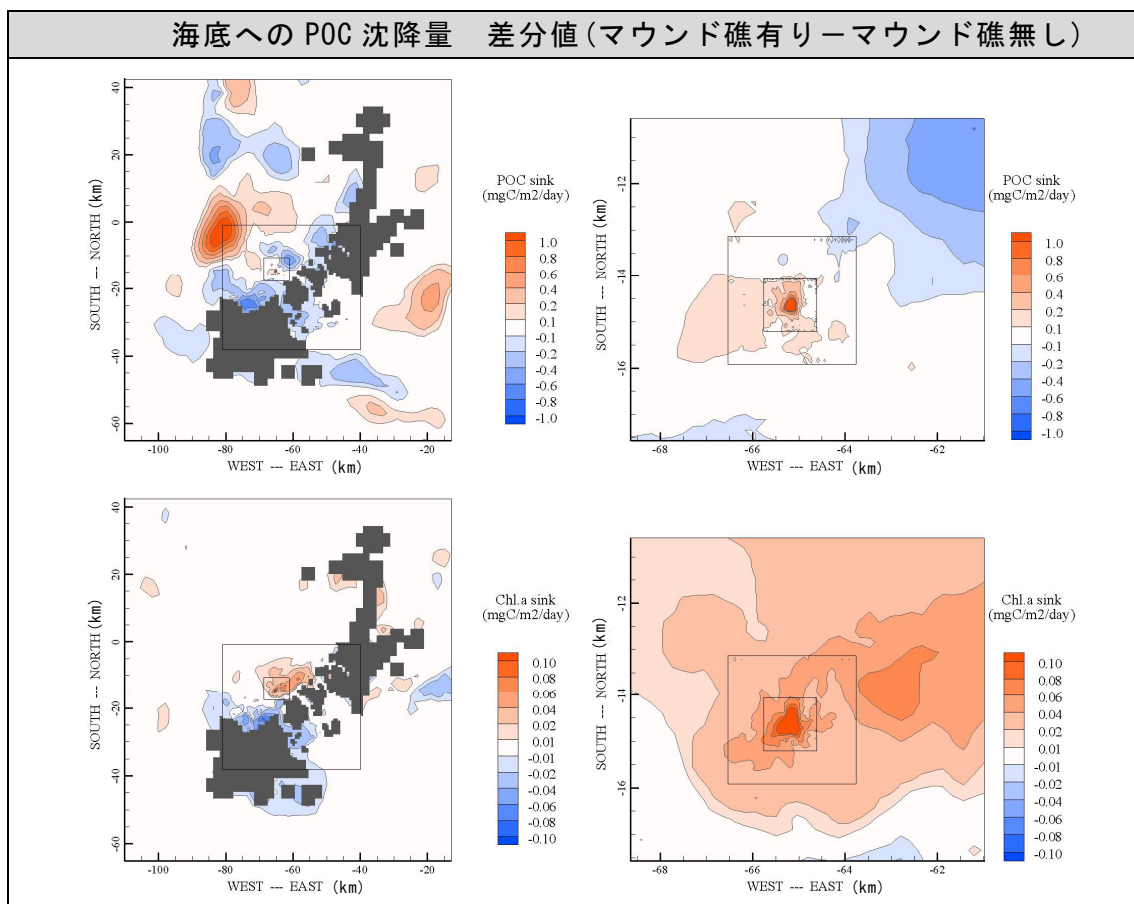
図VI-4. 3. 14 海底への POC 沈降量差分値 (マウンド礁有リーマウンド礁無し)
