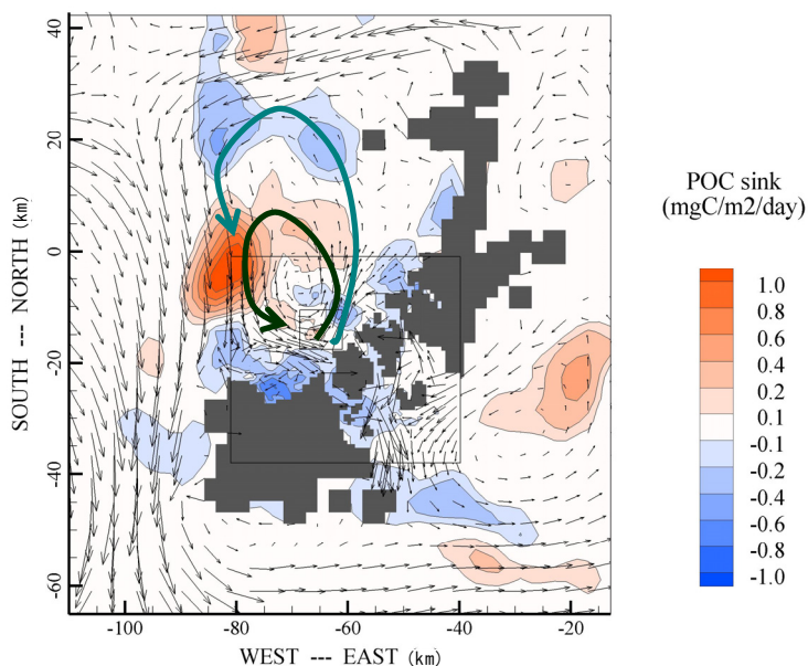
図VI-4.3.16 海底への全 POC 沈降量の分布
