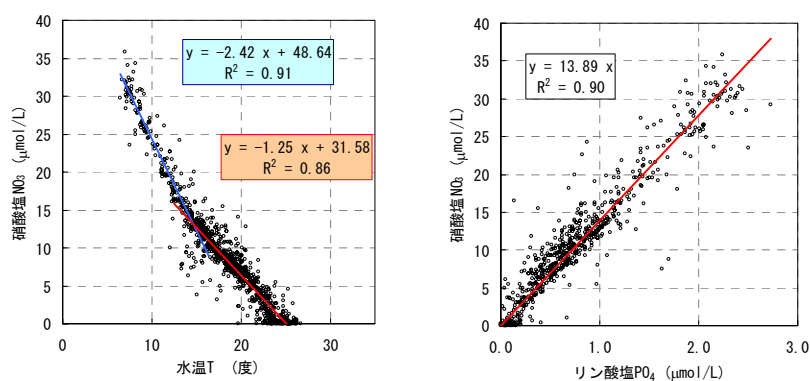
図VI-4.3.6 水温- \text{NO}_3 相関図(左図)および \text{NO}_3 - \text{PO}_4 相関図(右図)
