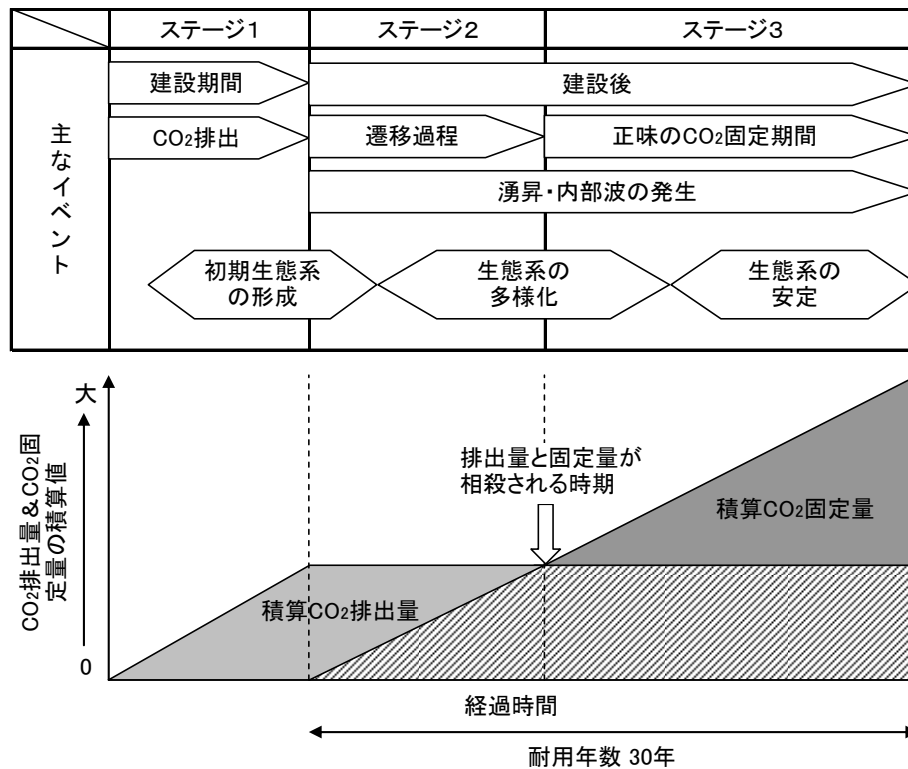
図 VI-1.1 湧昇マウンド礁による CO 2 固定効果の概念図
