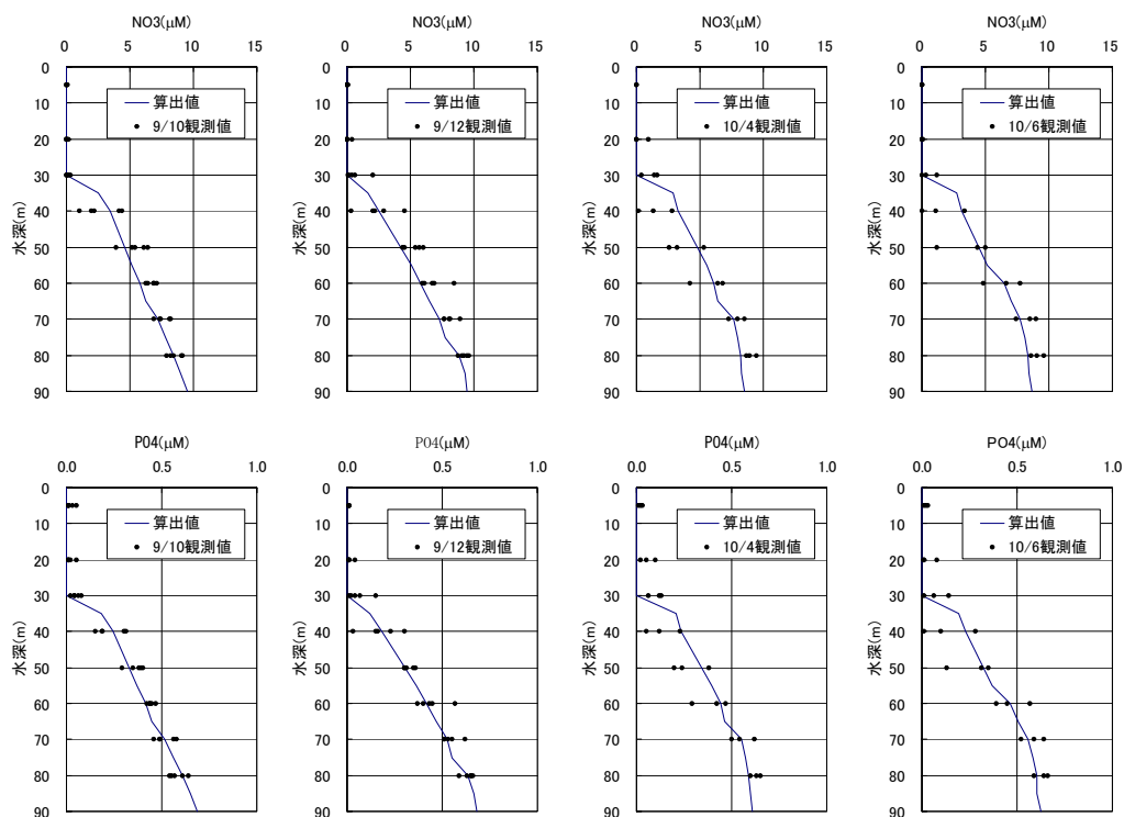
図VI-4.3.7 調査結果と水温からの栄養塩( \text{NO}_3 , \text{PO}_4 )算出結果の比較図
