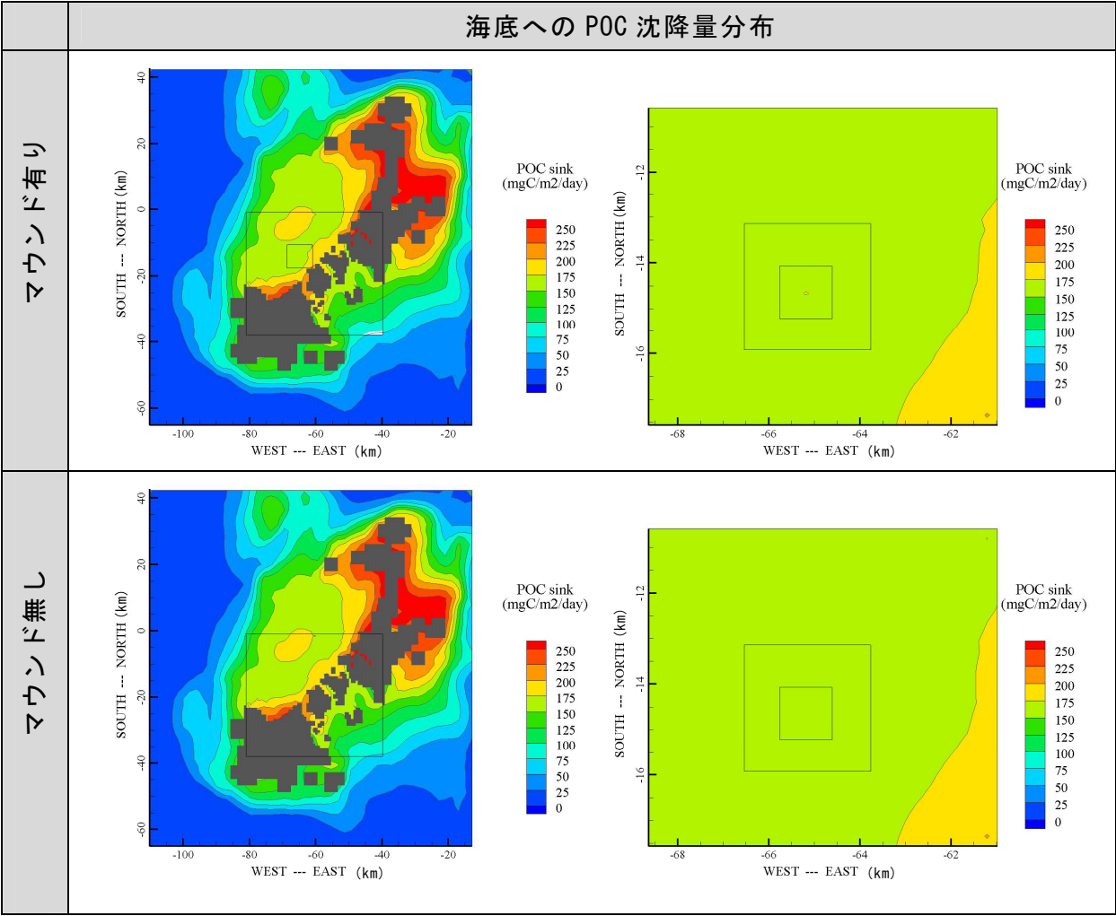
図VI-4.3.13 海底への全 POC 沈降量分布図(計算期間平均)
